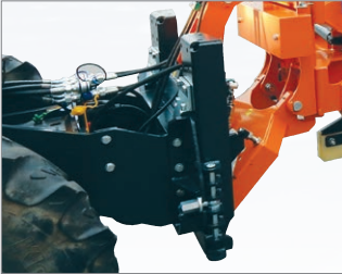
Kommunale Anbauplatte
